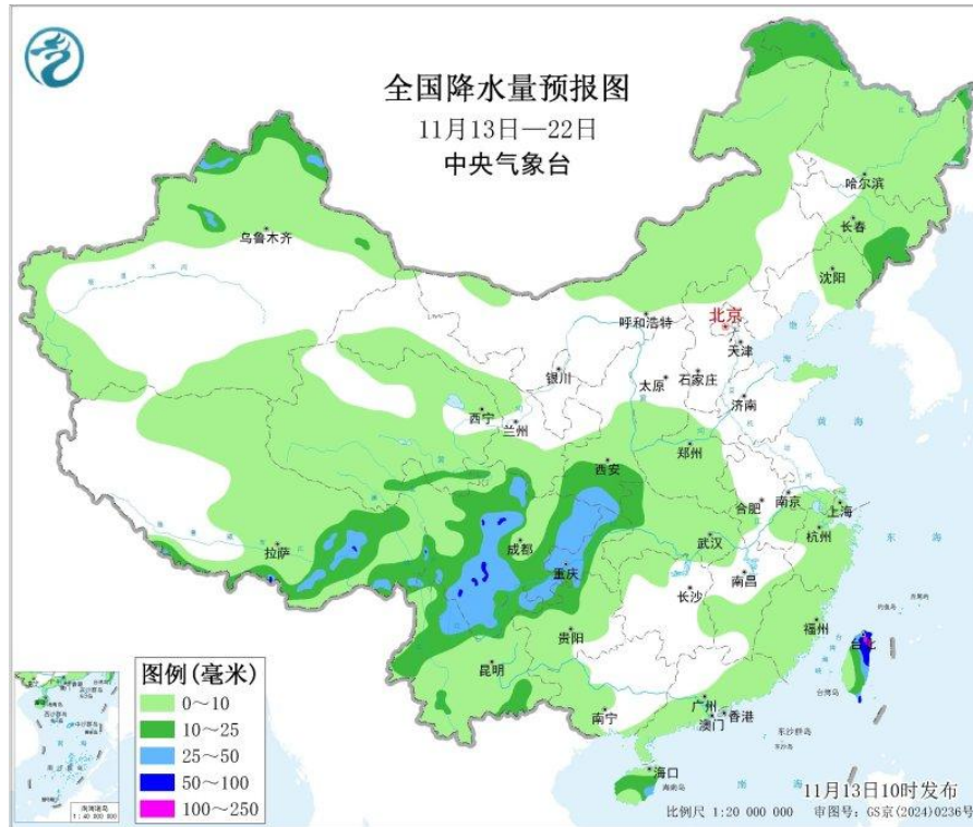
图 14 全国降水量预报图
